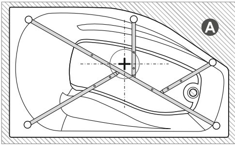
A* Размещение ножки. Ванна «Venta» левая. Tabanyn omalastyry. «Venta» akril shomylygysy sol jaq.
