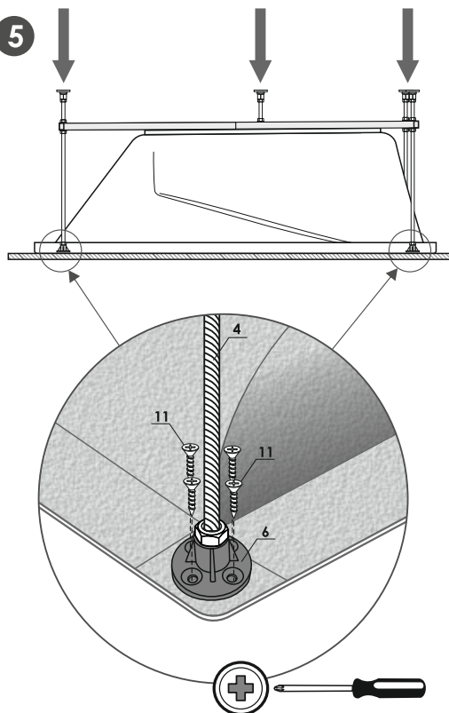
A* Размещение рамы. Ванна «Venta» левая. Jaqtayyn ornalastyry. «Venta» akril shomylygysy sol jaq.
