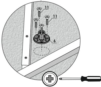
B* Размещение ножки. Ванна «Venta» правая. Tabanyn omalastyry. «Venta» akril shomylygysy oñ jaq.
