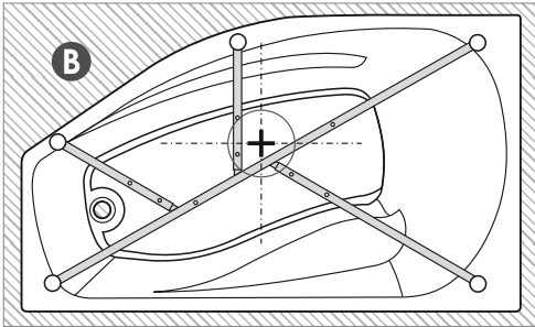
B* Размещение ножки. Ванна «Venta» правая. Tabanyn omalastyry. «Venta» akril shomylygysy oñ jaq.
