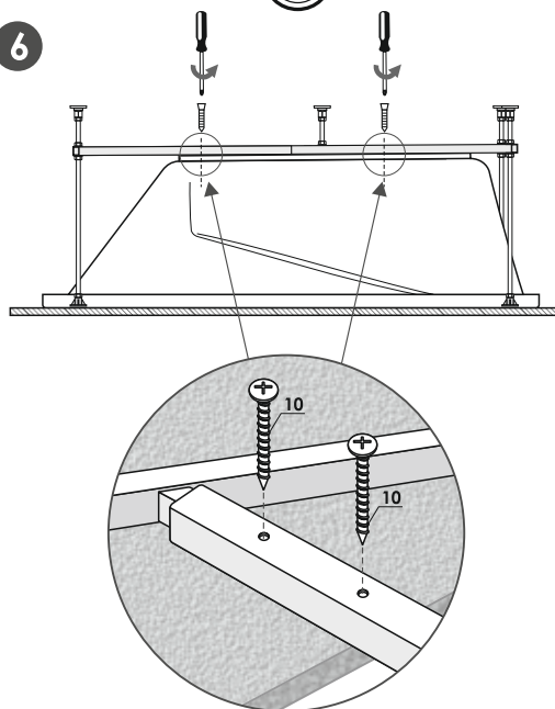
B* Размещение рамы. Ванна «Venta» правая. Jaqtayyn ornalastyry. «Venta» akril shomylygysy oň jaq.
