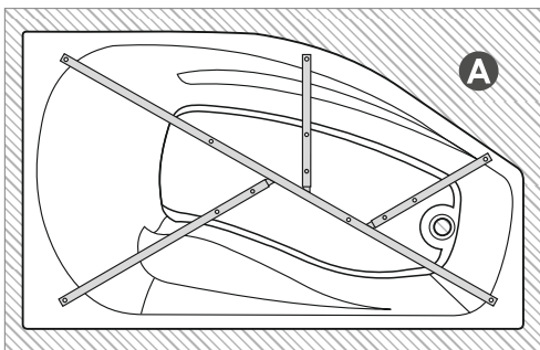
A* Размещение рамы. Ванна «Venta» левая. Jaqtayyn ornalastyry. «Venta» akril shomylygysy sol jaq.
