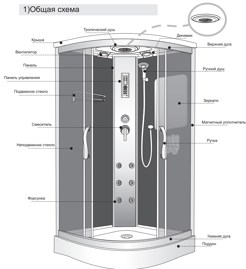
Общий вид душевой кабины
