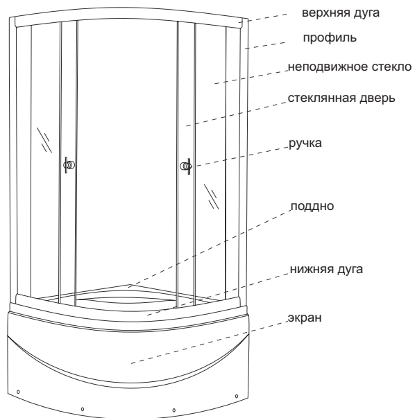
Конструкция кабины
