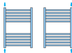
Схема 3 Подключение вертикальное
